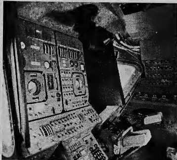
Un bista den interior di e Model Lunar di Excursion ta muestra e gran cantidad di instrumento y equipo cu e astronautanan lo tin cu traha cune. Diseño di e vehiculo ta compatible cu e exigencianan astronautica mientras nan ta riba luna.
